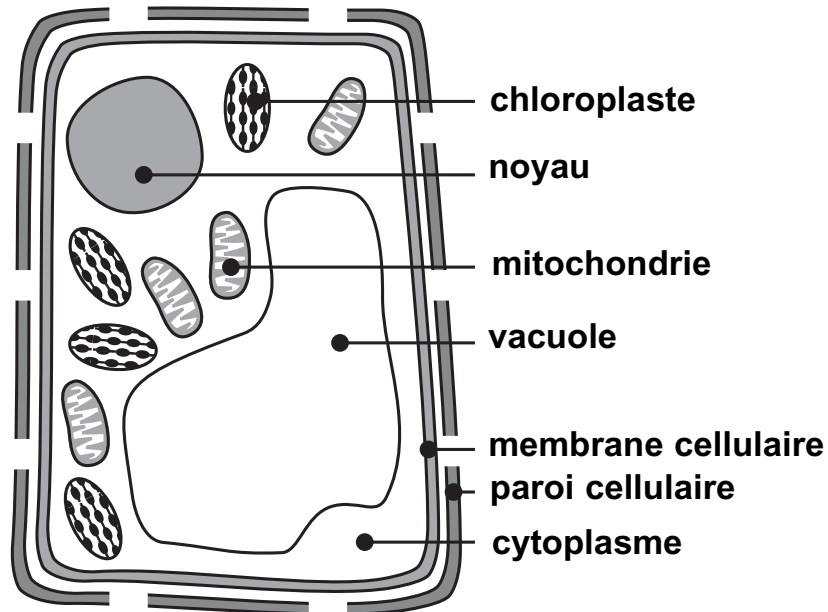
Diagramme simplifié d'une cellule végétale
